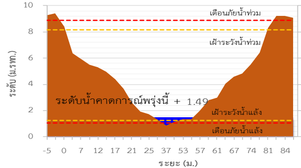
TC220605 สะพานตำรง
